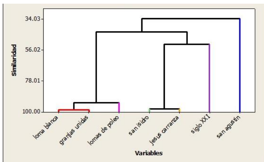
Figura 6. Dendrograma de correlaciones entre las distintas localidades.
