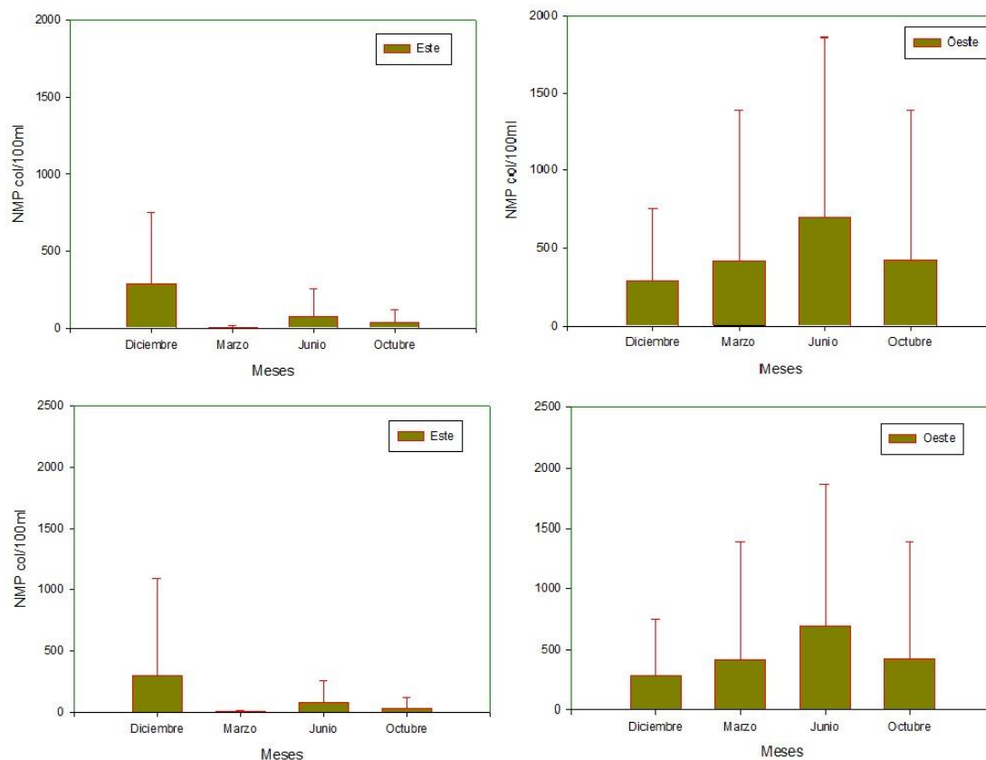
Figura 3. Comparación zona Este y Oeste por Fermentación por Tubos Múltiples coliformes totales (parte superior) y coliformes fecales (parte inferior).
