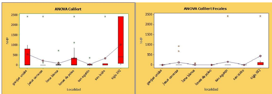
Figura 4. ANOVA Colilert para coliformes totales (Izquierda) y coliformes fecales (derecha).
