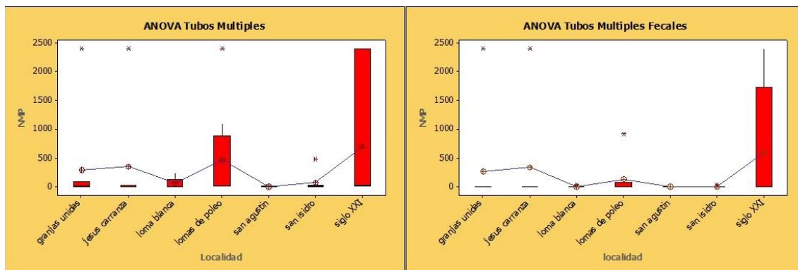
Figura 2. ANOVA fermentación por fermentación por tubos múltiples para coliformes totales (izquierda) y coliformes fecales (derecha).
