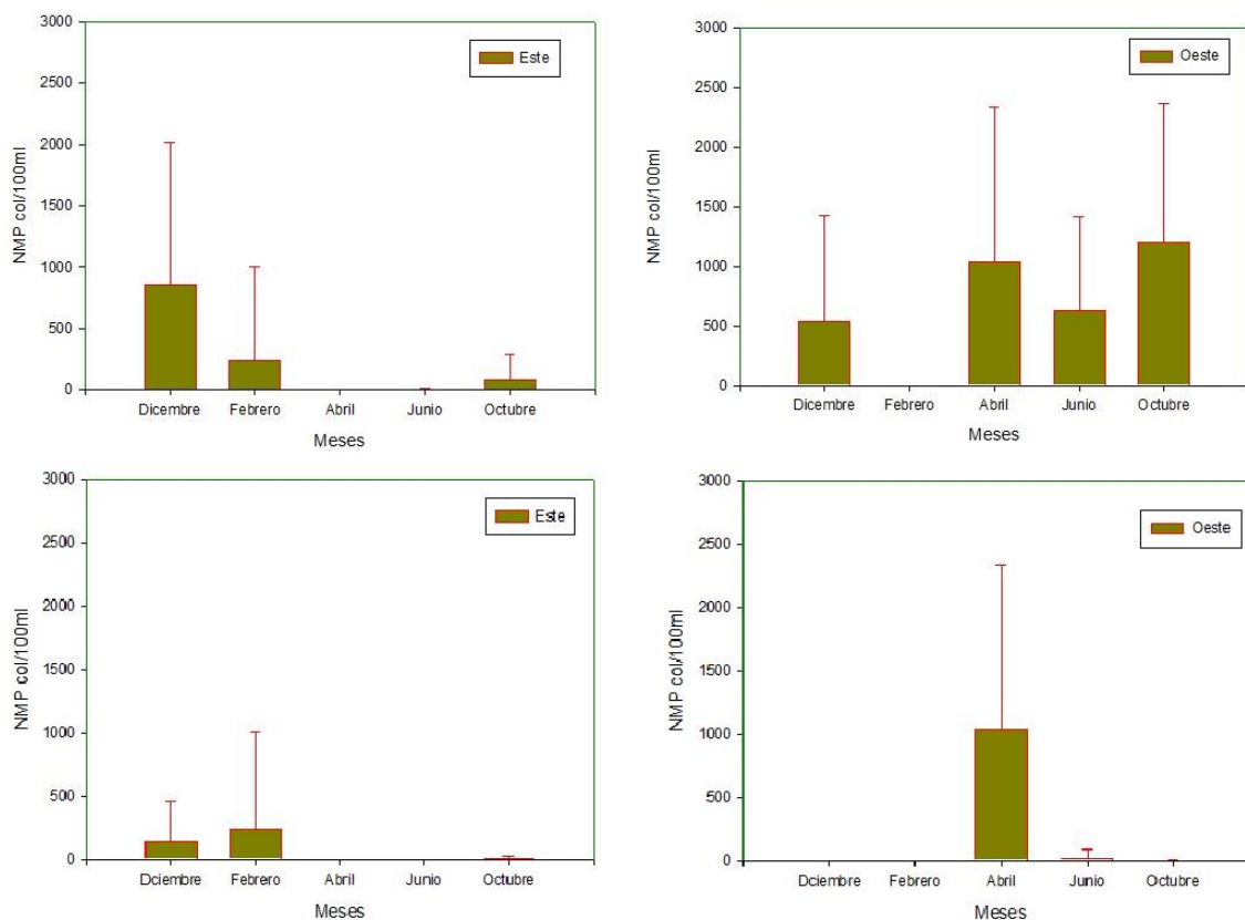
Figura 5. Comparación zona Este y Oeste por autoanálisis Colilert de coliformes totales y coliformes fecales.
